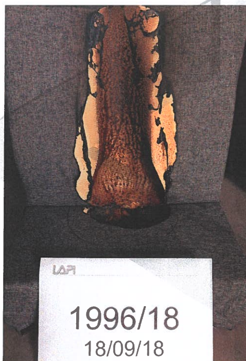
Foto 2: dopo la prova / Picture 2: after testing
